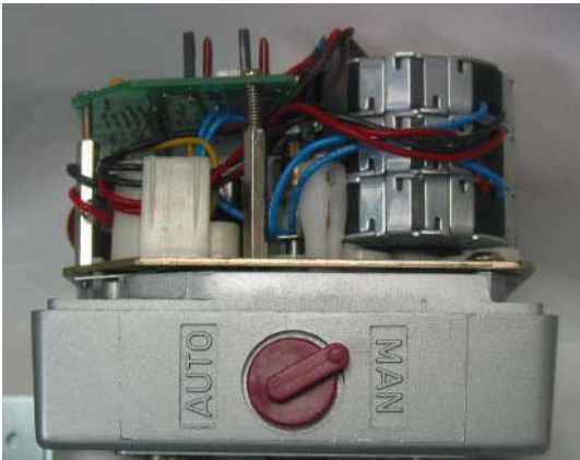
수동/자동 노브 auto/manual knob
