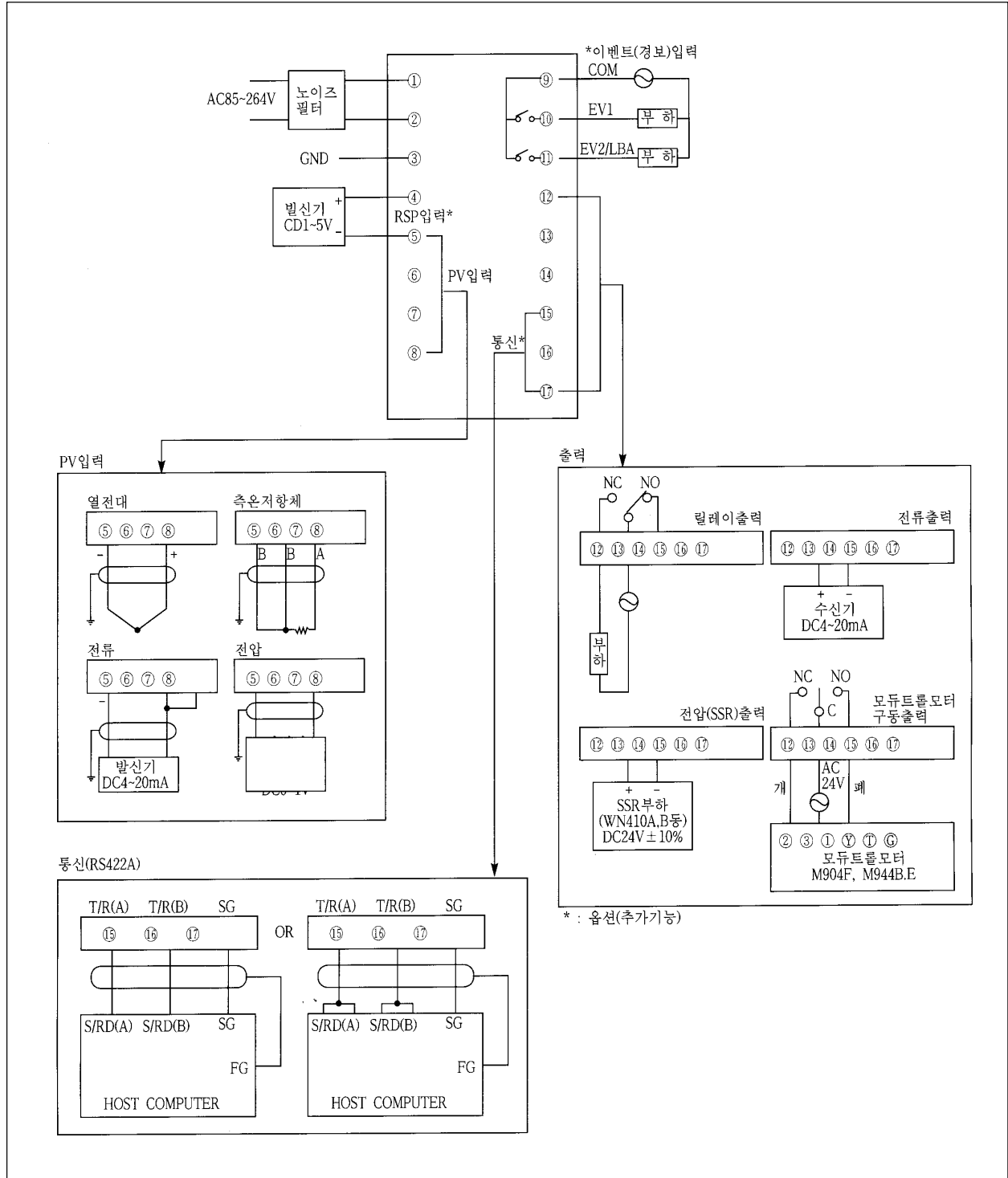
그림 3. 결선도
